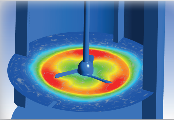
CFD SİMÜLASYON HWM KARIŞTIRMA TANKI
